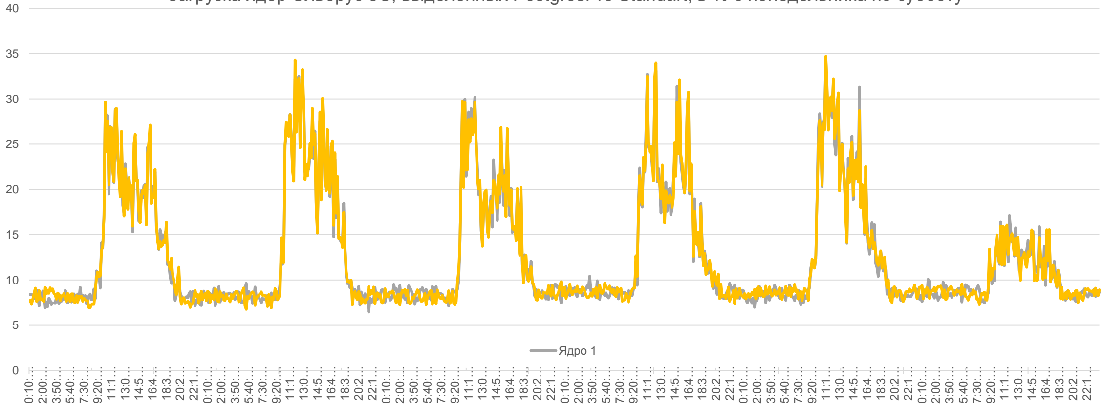
Загрузка ядер Эльбрус 8С, выделенных PostgresPro Standart, в % с понедельника по субботу
